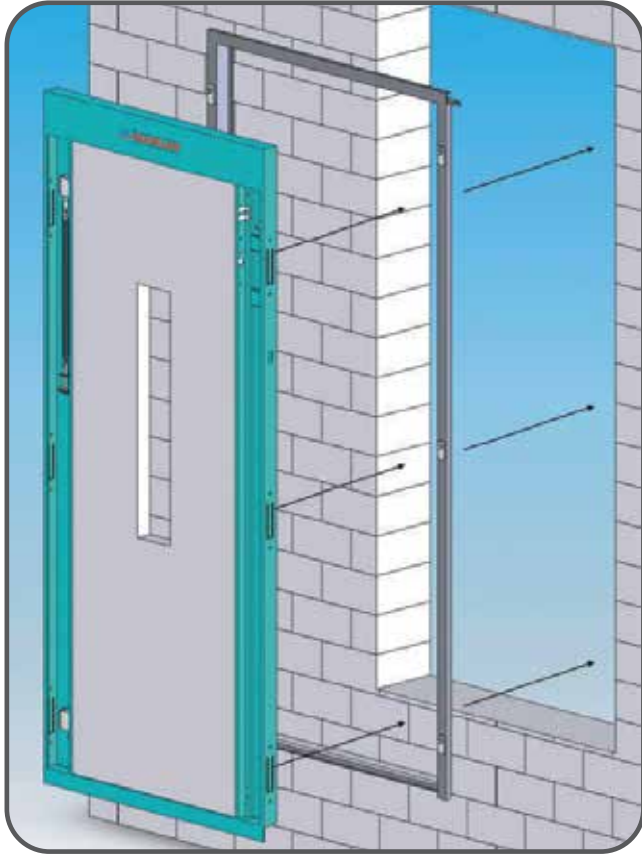
ŞEKİL - 1 Körkasalı Montajı / Mounting With Subframe
