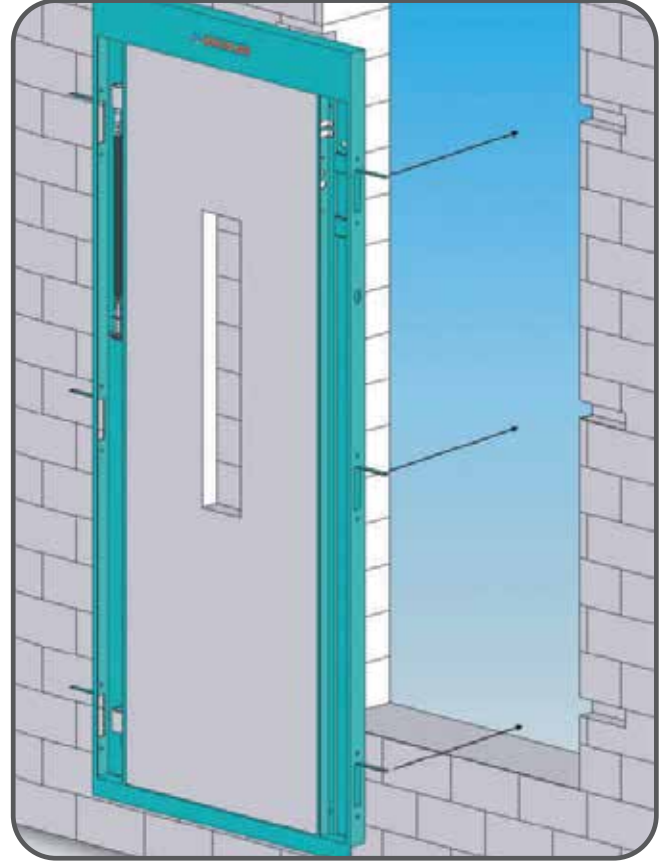
ŞEKİL - 2 Körkasasız Montajı / Mounting Without Subframe
